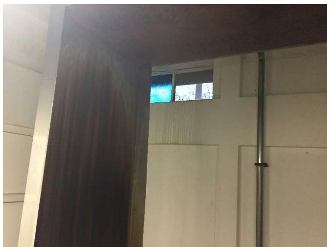
Figur 5. Udluftning i rummet sker gennem insektnet. Ved tilsynet i januar 2020 var anlægget ikke i drift.
