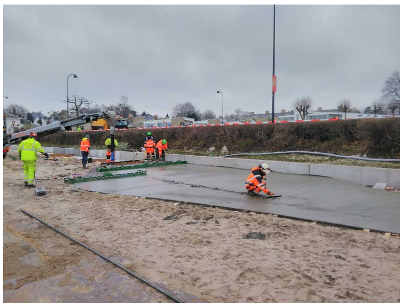
Stiforløbet anlægges.
