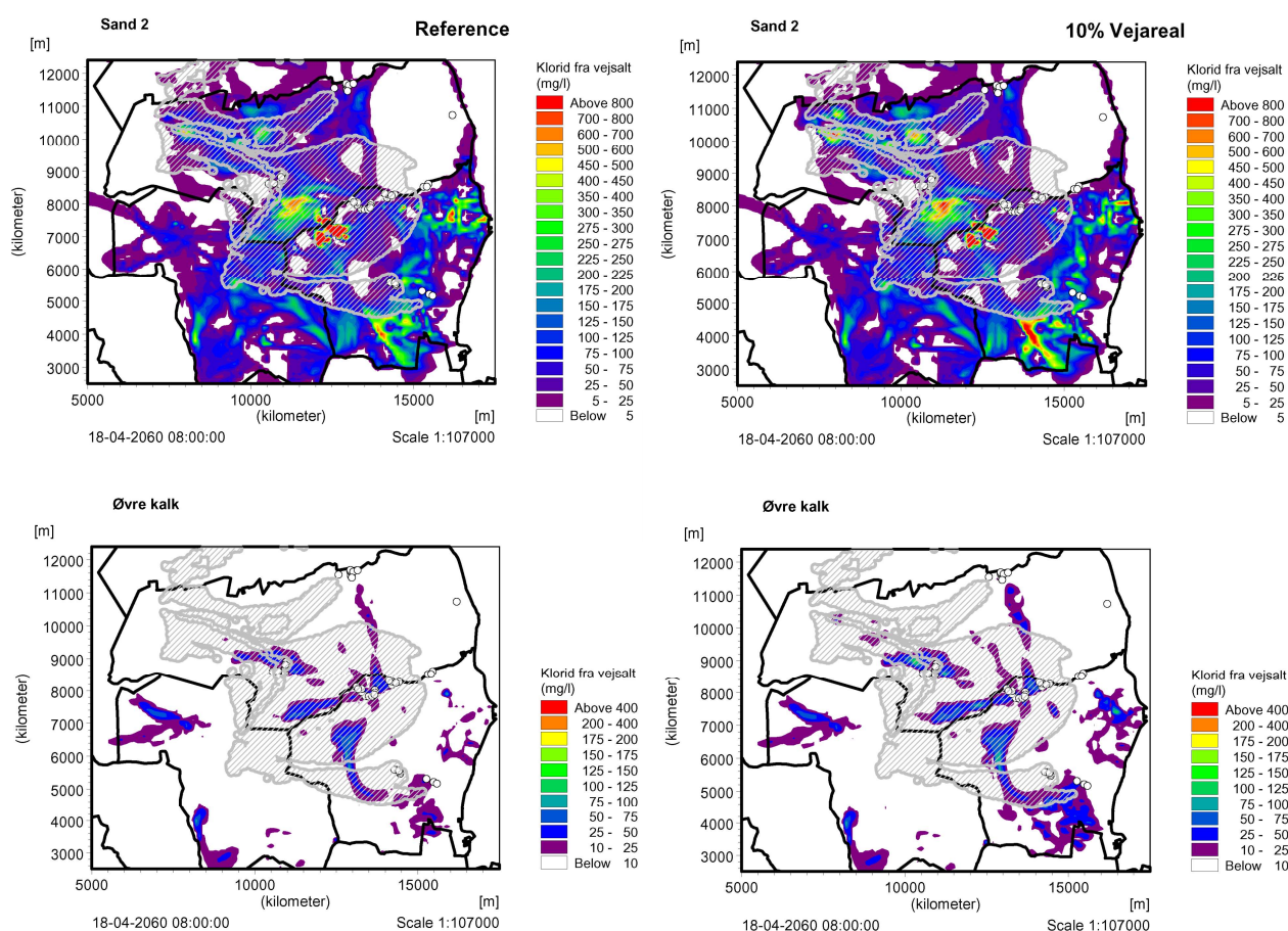
Figur 5. Sammenligning af klorid fra vejsalt i 2060 for reference scenarium 1 (venstre) og scenarium 4 (højre) vist for Sand2 magasinet (øverst) og kalk magasinet (nederst).
